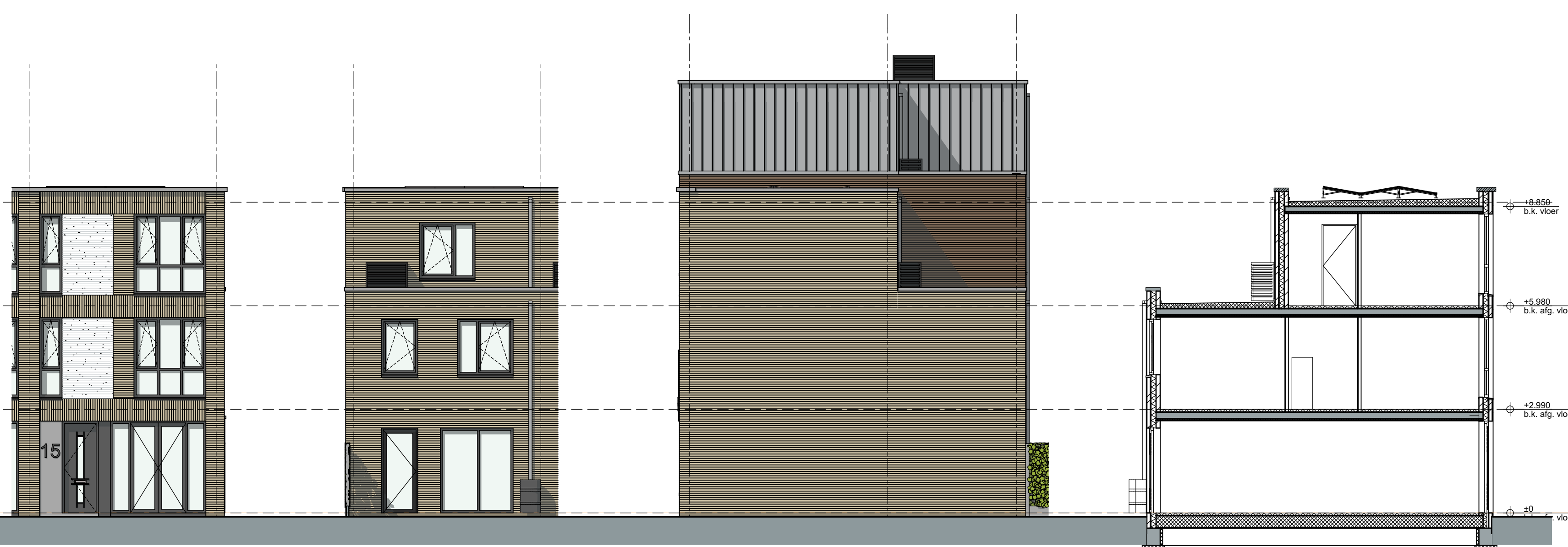
Voorgevel West
